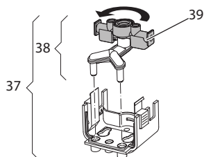
Рис. 21: Поворот впускного отверстия
